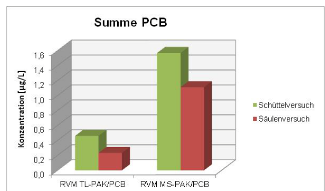
Abb. 4: Vergleich Säulen- und Schüttelverfahren PCB
