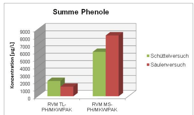
Abb. 3: Vergleich Säulen- und Schüttelverfahren Phenole
