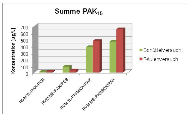
Abb. 1: Vergleich Säulen- und Schüttelverfahren PAK
