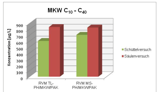
Abb. 2: Vergleich Säulen- und Schüttelverfahren MKW
