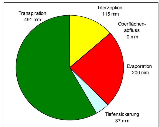
Abb. 1: Anteile der Wasserbilanzkomponenten für die Buchenfläche im Mittel der Jahre 1961 – 1990.
