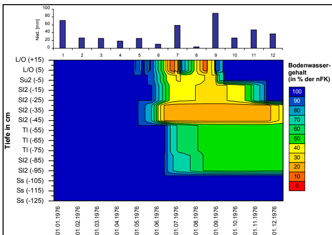
Abb. 2: Entwicklung des pflanzenverfügbaren Bodenwassers im Trockenjahr 1976 am Beispiel der Buchenfläche (Monatsniederschläge als Balkendiagramm)
