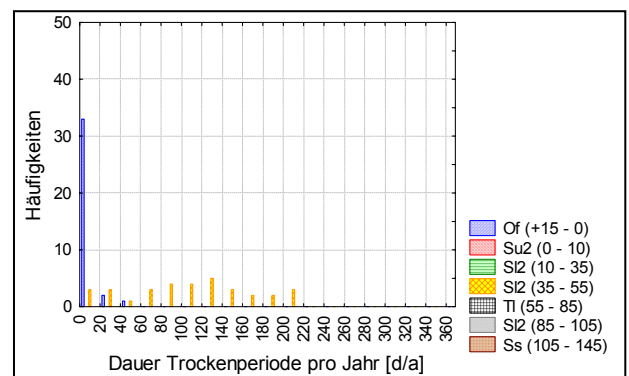
Abb. 3: Häufigkeiten von Trockenperioden (BWG < 40 % der nFK) bei Annahme des Szenarios A1B trocken, Buche mit forstlicher Nutzung, 2021 – 2050
