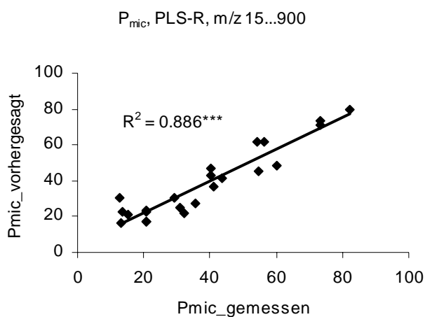
Abb. 1: Korrelation zwischen den mittels Massenspektrometrie vorhergesagten und mittels Fumigations-Extraktionsmethode gemessenen P_{mic} Gehalten ( \text{mg kg}^{-1} ) des Bodens
