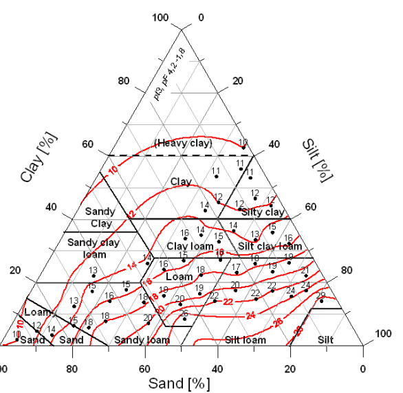
Abbildung 2: Poren 0,2 - 50µm, nutzbare Feldkapazität (Vol.-%) (Trockenrohdichte 1,4-1,6 g/cm 3 )
