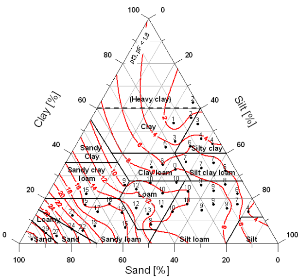
Abbildung 1: Poren > 50µm, Luftkapazität (Vol.-%) (Trockenrohdichte 1,4-1,6 g/cm 3 )
