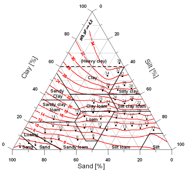
Abbildung 4: Poren < 0,2\mu\text{m} , Totwasser (Vol.-%) (Trockenrohdichte 1,4-1,6 \text{g/cm}^3 )
