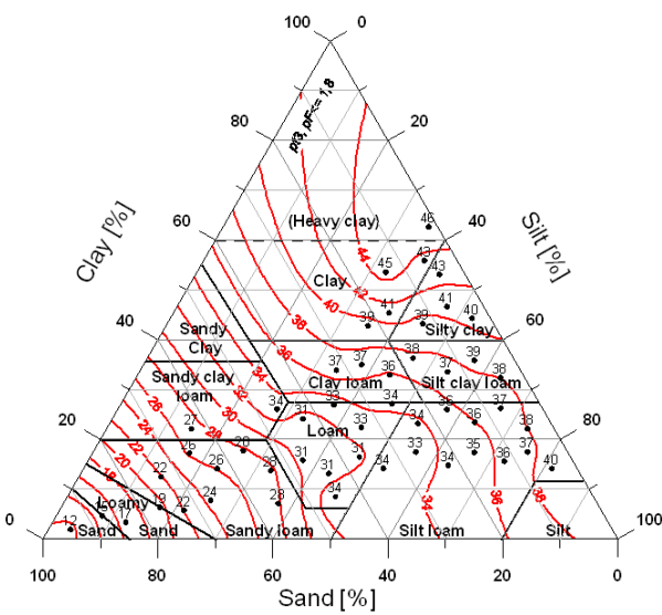
Abbildung 3: Poren \leq 50 \mu\text{m} , Feldkapazität (Vol.-%) (Trockenrohdichte 1,4-1,6 \text{g/cm}^3 )
