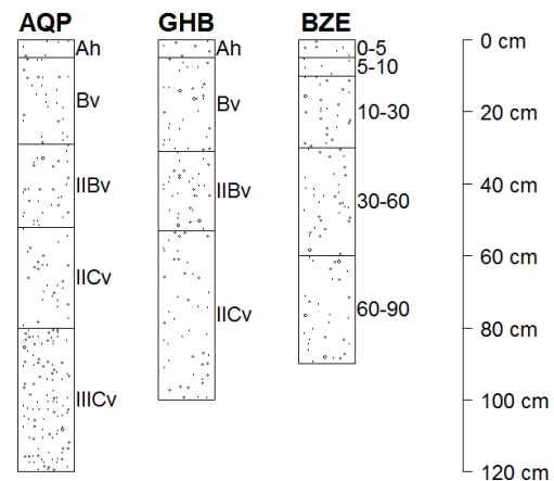
Abb. 1 Leitprofile für die drei verschiedenen Aggregierungsansätze AQP – Aggregation entlang eines kontinuierlichen Tiefenverlaufes, GHB – separate Aggregation Generalisierter Horizontbezeichnungen, BZE – Aggregation über die Tiefenstufen der BZE II.
