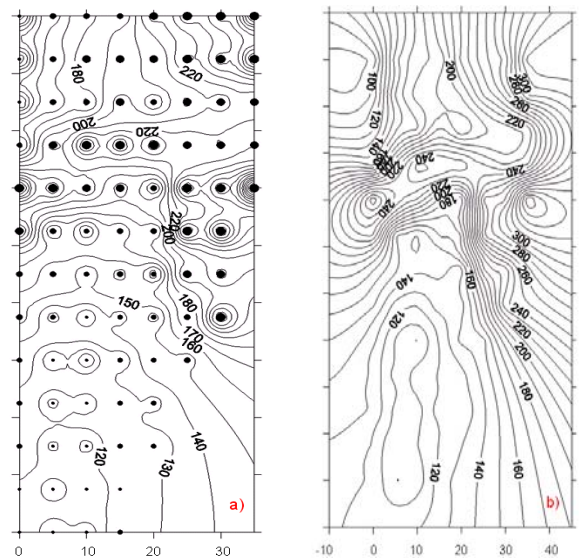
Abb. 5: Zink-Verteilung (a) und Kriging-Extrapolation (b)
